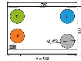
Vasenkätisen koneen mittakuva
