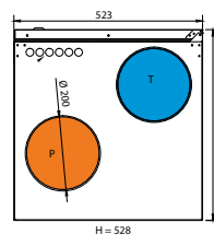
Oikea-/vasenkätisen koneen mittakuva
