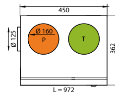
Oikeakätisen koneen mittakuva
