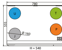
Oikeakätisen koneen mittakuva
