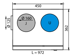
Vasenkätisen koneen mittakuva
