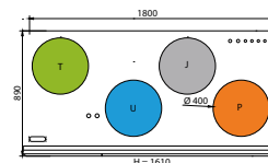
Vasenkätisen koneen mittakuva
