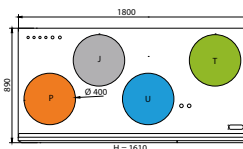
Oikeakätisen koneen mittakuva
