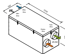
Oikea-/vasenkätisen koneen mittakuva
