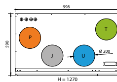
Oikeakätisen koneen mittakuva
