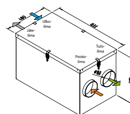
Oikeakätisen koneen mittakuva
