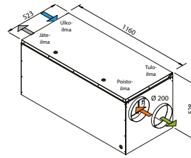
Oikea-/vasenkätisen koneen mittakuva
