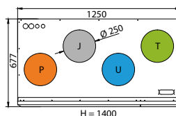
Oikeakätisen koneen mittakuva
