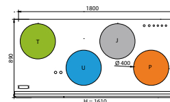
Vasenkäntisen koneen mittakuva
