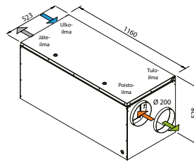
Oikea-/vasenkätisen koneen mittakuva
