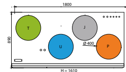
Vasenkätisen koneen mittakuva
