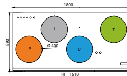
Oikeakätisen koneen mittakuva
