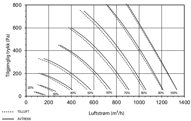
Kapasitetskurve for LTR-7 Z tillufts- og avtrekksvifte
