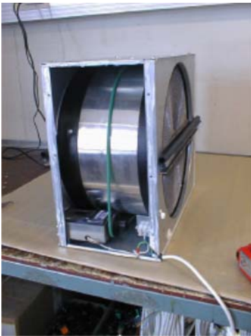
Bild 5 Värmeväxlaren (=rotorn) med drivremmen monterad
