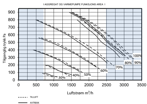
Kapasitetskurve for Pallas HP Aqua KI-W tillufts- og avtrekksvifter
