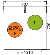
Oikea-/vasenkätisen koneen mittakuva
