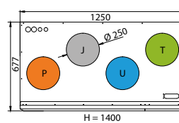
Oikeakätisen koneen mittakuva
