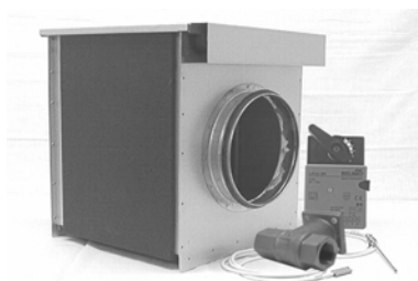
Lämmityspatteri, säätöventtiili, venttiilitoimilaite, kanavalämpötila-anturi, vesipatterin jäätymissuoja-anturi (ACW-mallit)
