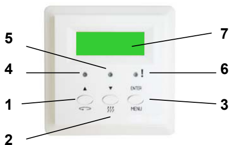
LTR-3-AC ohjainpaneeli
