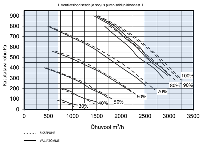
Pallas HP Aqua KI-W sissepuhe ja väljatõmme tunnusjooni koos F7/M5 filter
